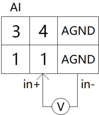
图 2.8 PLC-221 AI 接线
