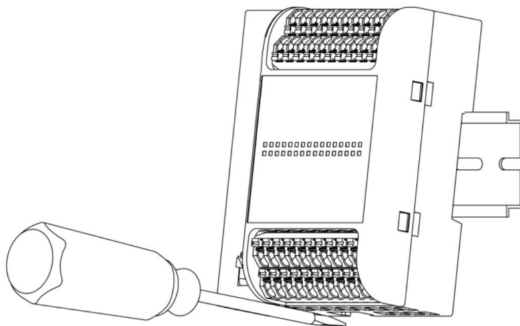
图 2.3 GCAN-PLC-221 CANopen 模块拆卸
