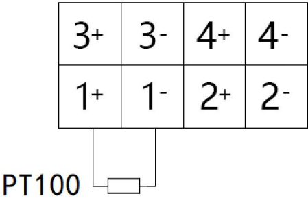
图 2.9 PLC-221 PT100 接线
