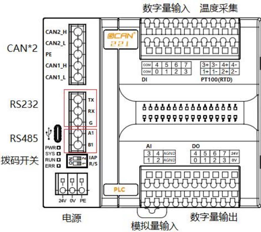
图 2.4 PLC-221 各接口位置
