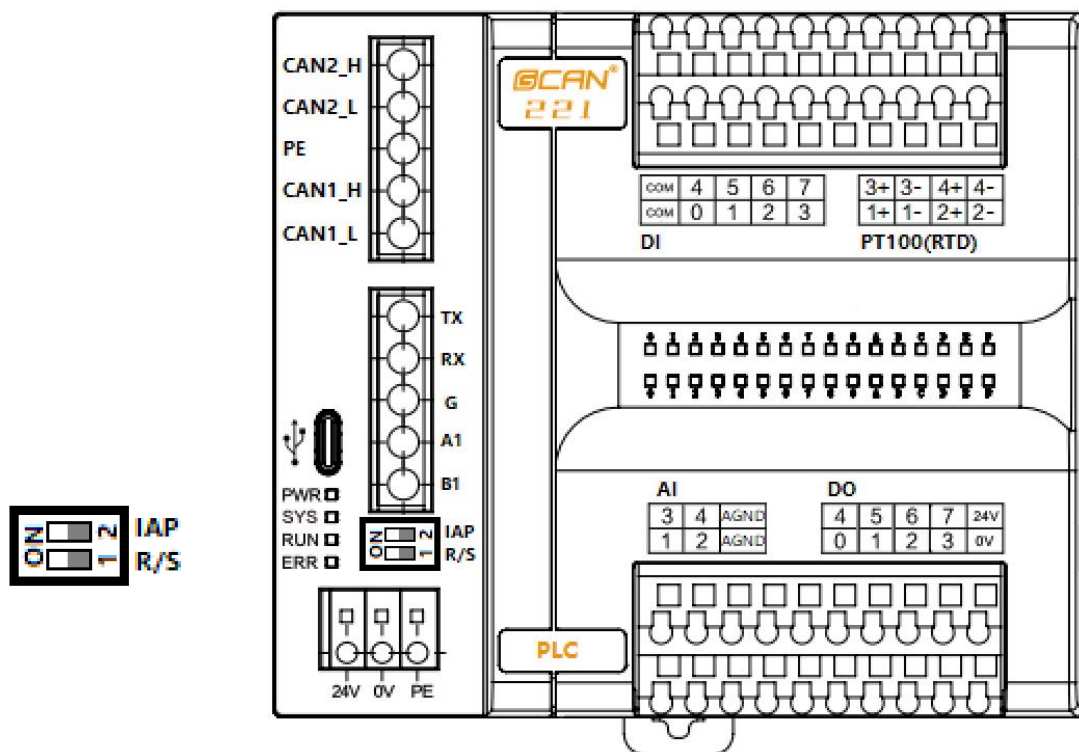
4.1 GCAN-PLC-221 拨码开关图
