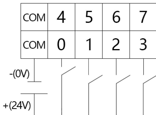
图2.7 PLC-221 DI (0-3路) 源型接线
