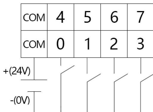
图 2.6 PLC-221 DI (0-3 路) 漏型接线
