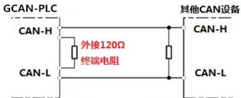
图 3.3 GCAN-PLC-221 与其他 CAN 节点设备连接
