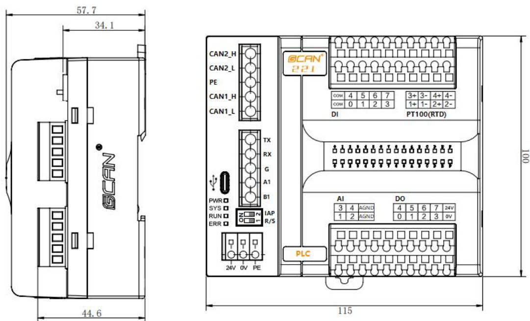
图 2.1 GCAN-PLC-221 模块外形尺寸图
