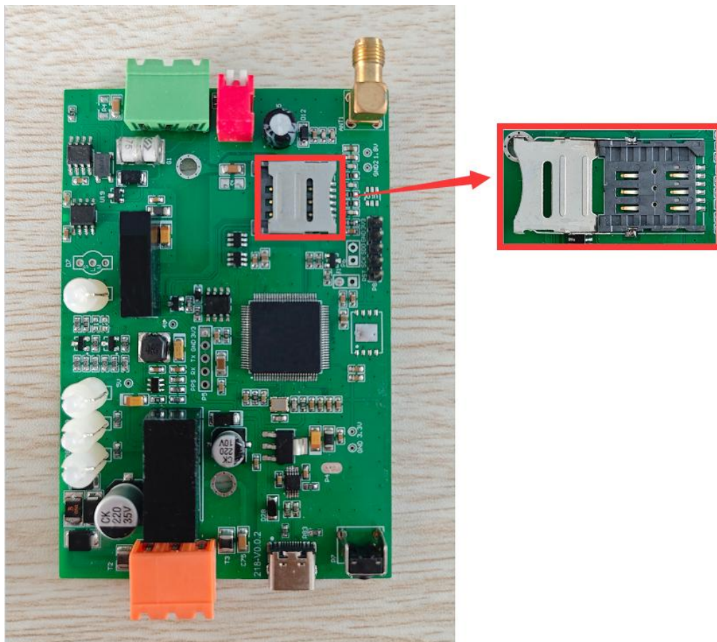
图 3.1 4G 卡安装位置
