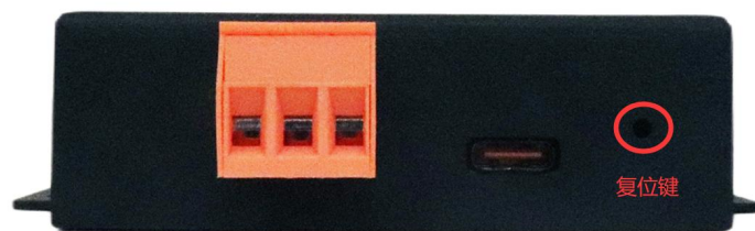
图 2.3 电源及其他接口位置
