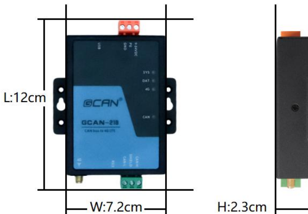
图 2.1 GCAN-218 外形尺寸
