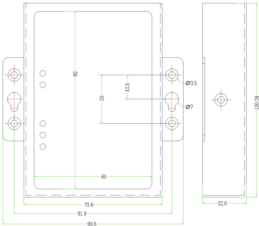
图 2.2 GCAN-218 安装尺寸
