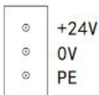
图 2.9 GCAN-PLC-301/302 的电源端子排
