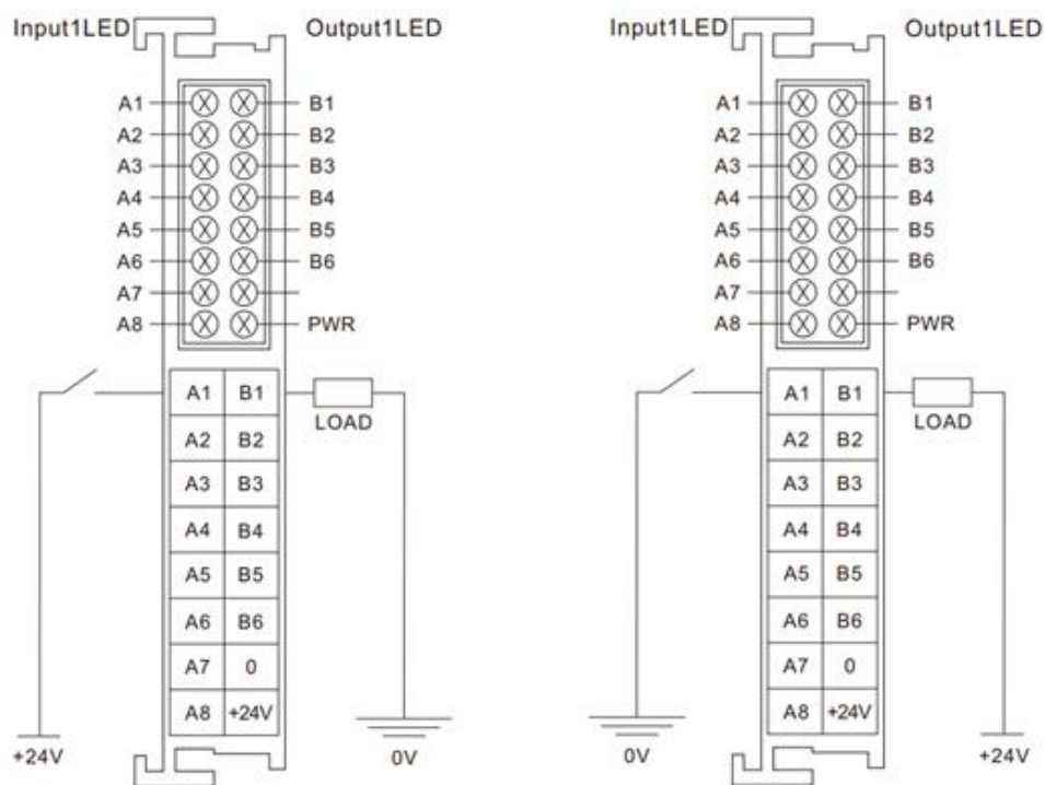
图 2.10 PNP 型接线端子排
