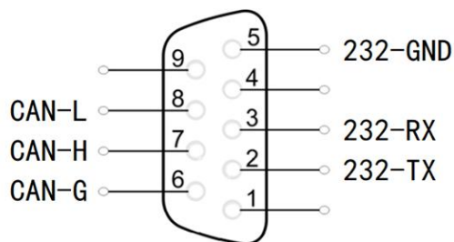
图 2.7-2 GCAN-PLC-302 接口定义
