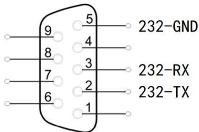
图 2.7-1 GCAN-PLC-301 接口定义
