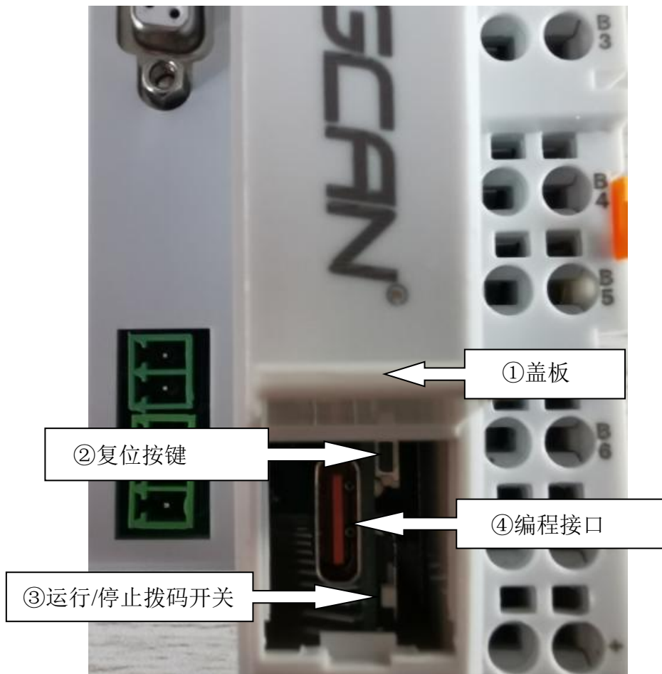
图 4.1 盖板打开后实物图
