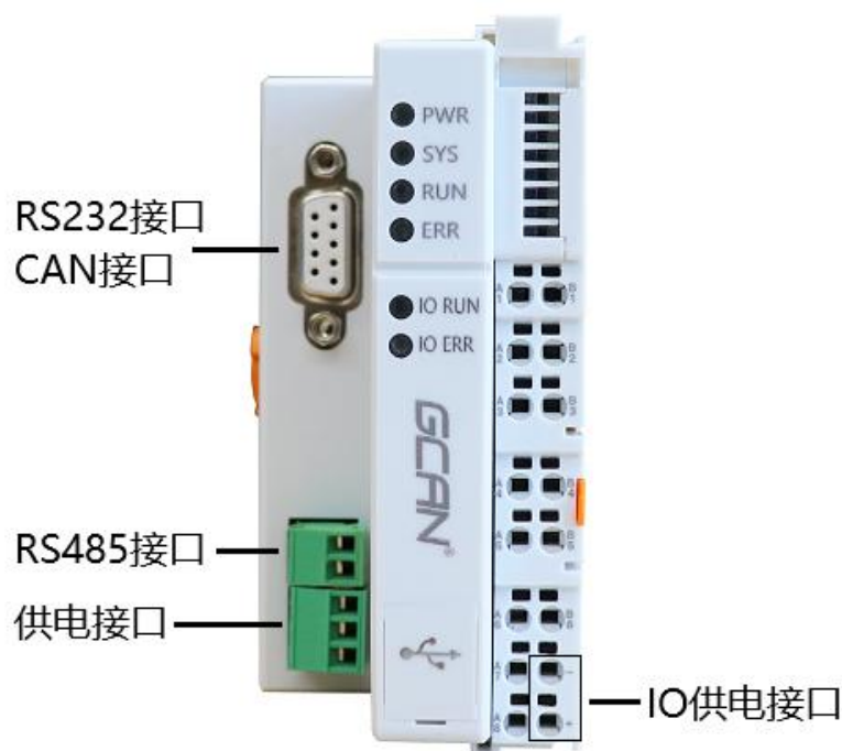
图 2.1 GCAN-PLC-302 外观接口图
