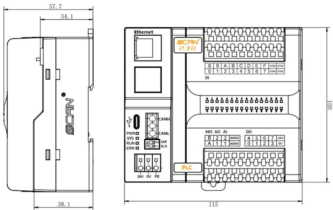
图 2.1 GCAN-PLC-230 模块外形尺寸图
