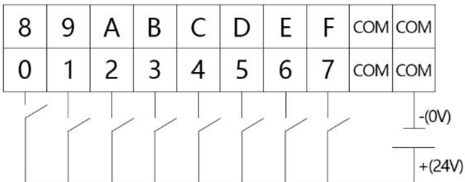
图2.7 PLC-230 DI（0-7路）源型接线
