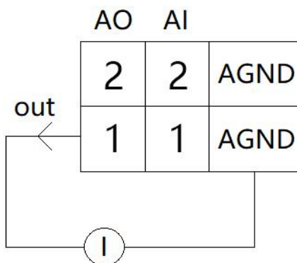
图2.8 PLC-230 AO接线
