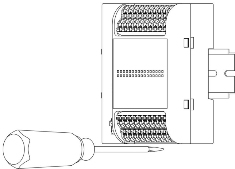
图 2.2 GCAN-PLC-230 CANopen 模块安装
