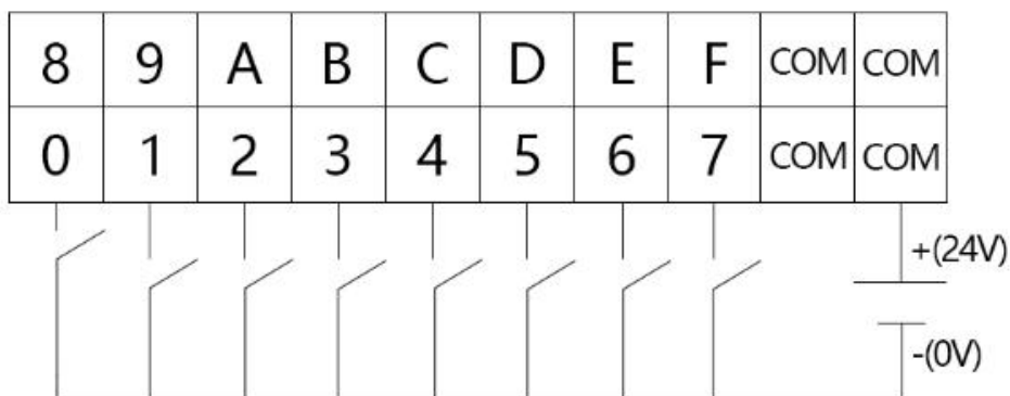
图 2.6 PLC-230 DI（0-7 路）漏型接线
