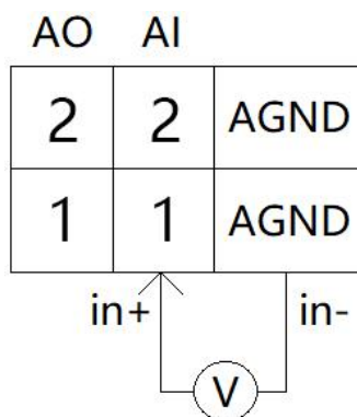
图2.9 PLC-230 AI接线
