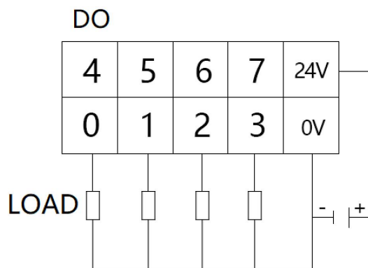
图 2.5 PLC-230 DO (0.1.2.3 路) 接线
