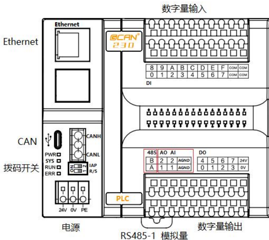
图 2.4 PLC-230 各接口位置
