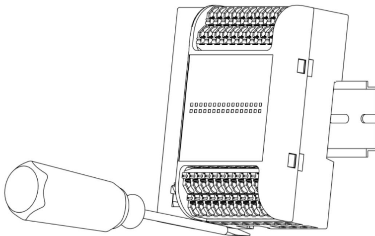
图 2.3 GCAN-PLC-230 CANopen 模块拆卸
