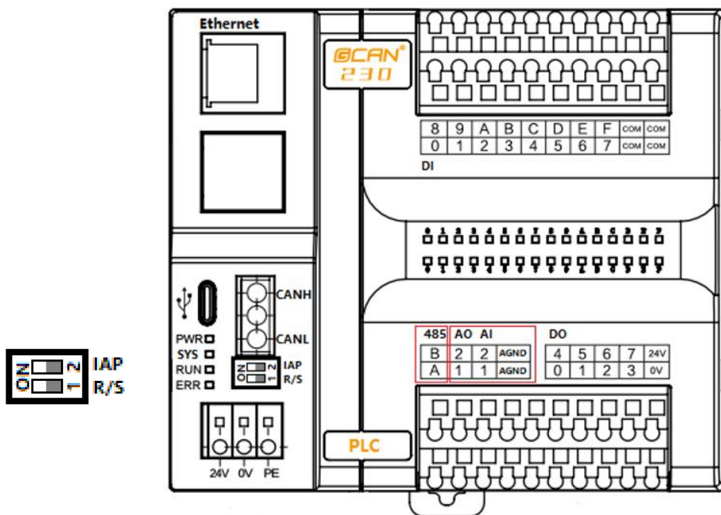
4.1 GCAN-PLC-230 拨码开关图
