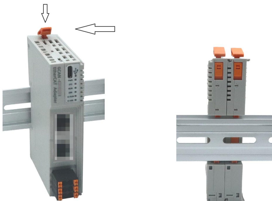
图 2.3 GCAN-PLC-325 可编程逻辑控制器模块安装
