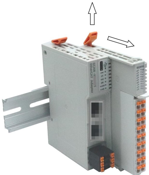
图 2.5 GCAN-PLC-325 可编程逻辑控制器拆卸
