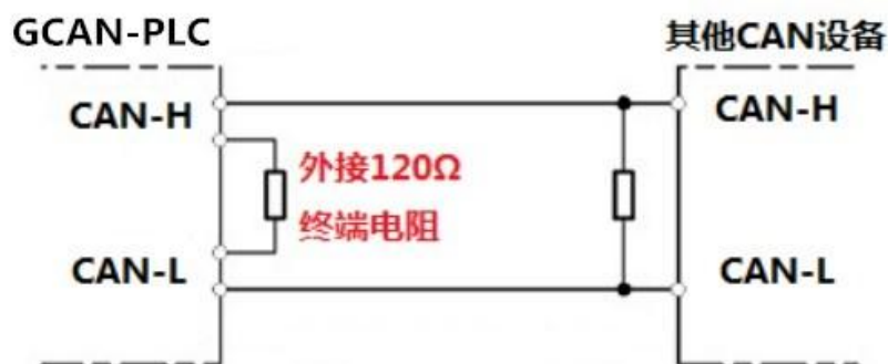
图 3.2 GCAN-PLC-325 与其他 CAN 节点设备连接
