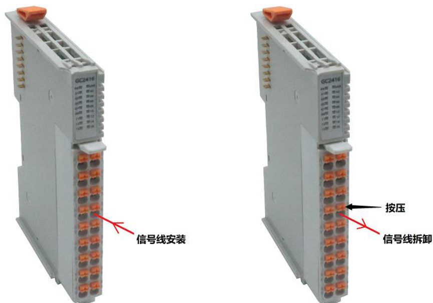
图 2.6 接线方法
