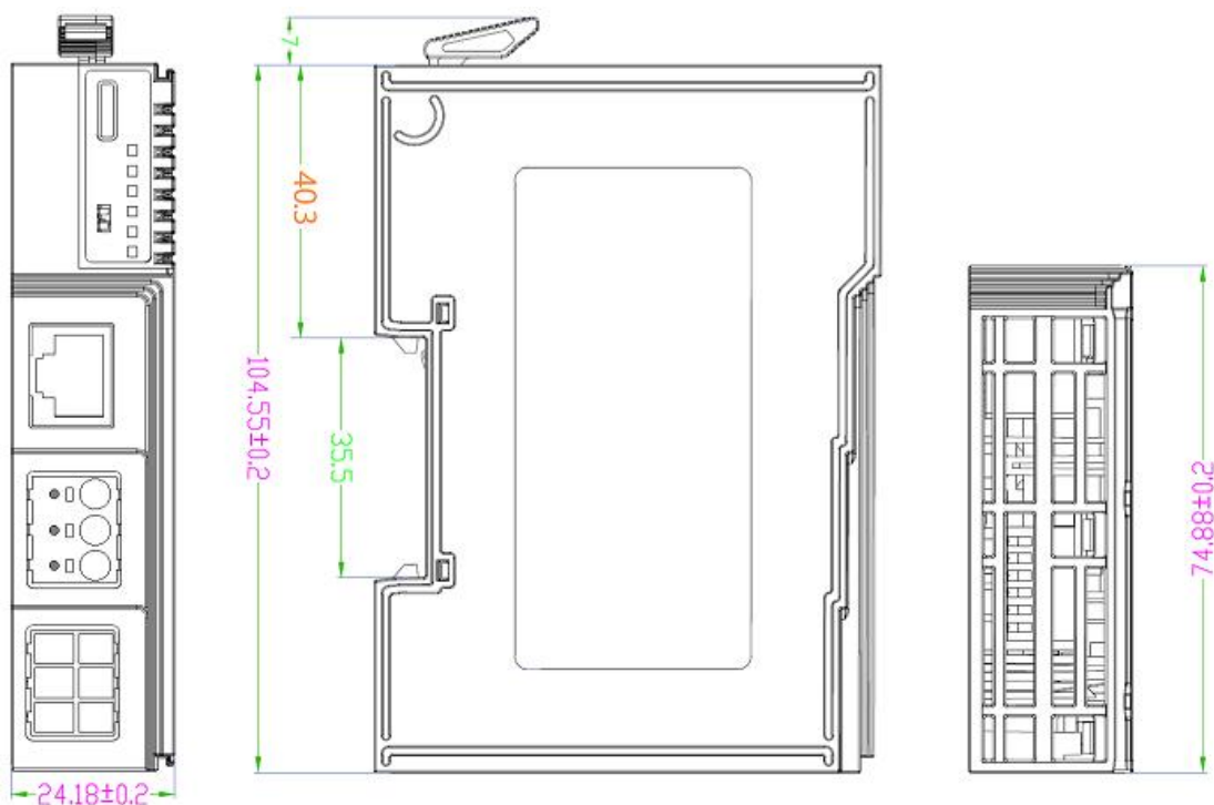
图 2.1 GCAN-PLC-325 可编程逻辑控制器外观及尺寸图
