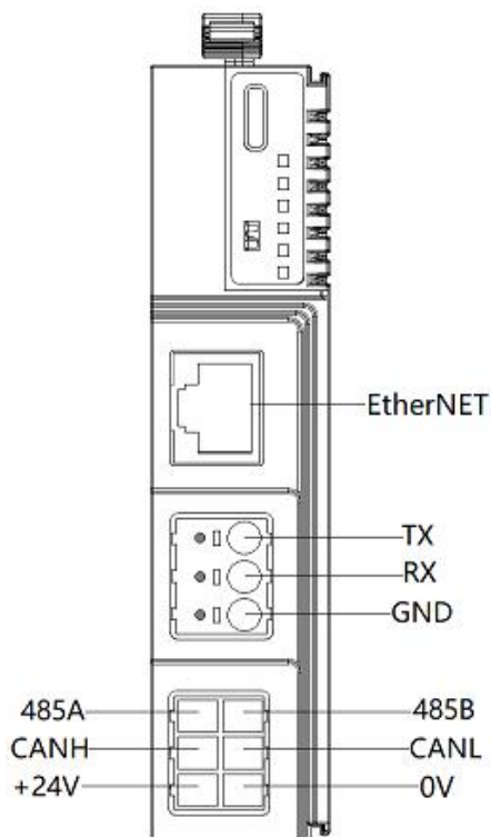
图 2.7 GCAN-PLC-325 总线及电源接线端子排
