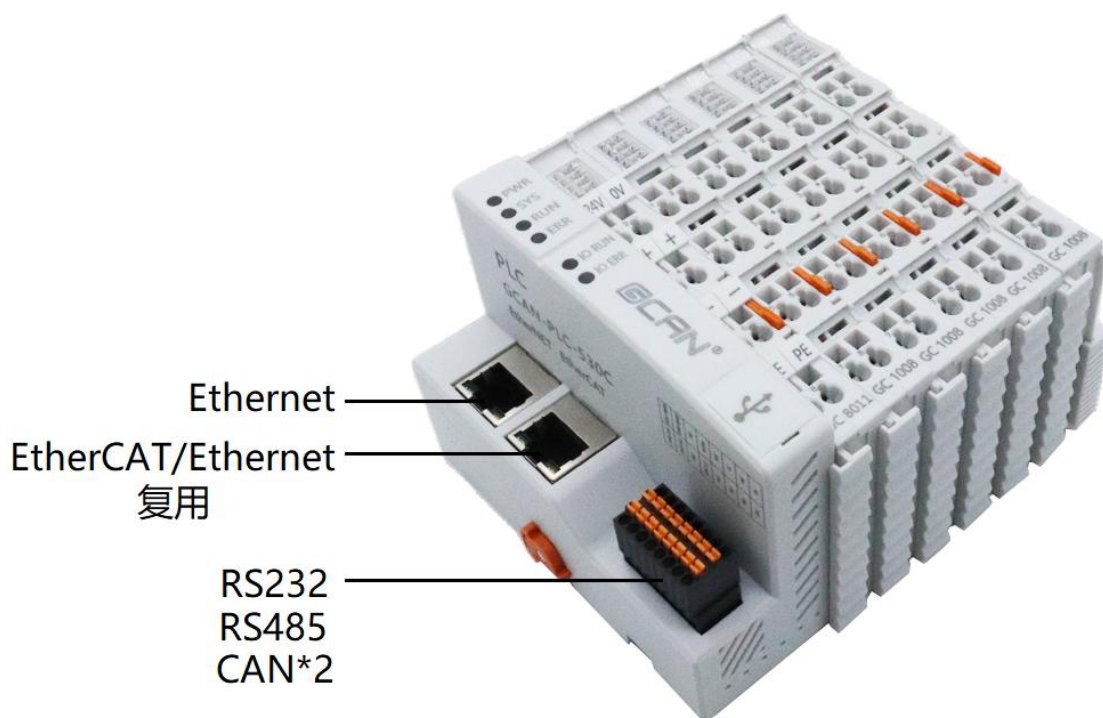
图 2.6 GCAN-PLC-530C 的总线接口样式
