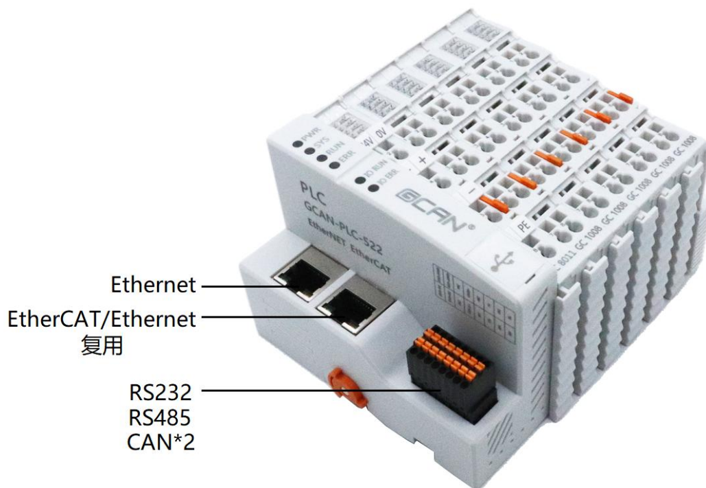
图 2.6 GCAN-PLC-522 的总线接口样式
