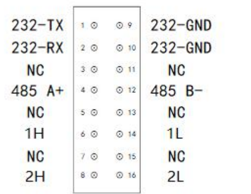
图 2.7 GCAN-PLC-522 的总线接口样式
