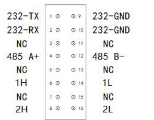
图 2.7 GCAN-PLC-521 的总线接口样式
