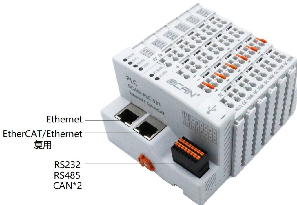
图 2.6 GCAN-PLC-521 的总线接口样式
