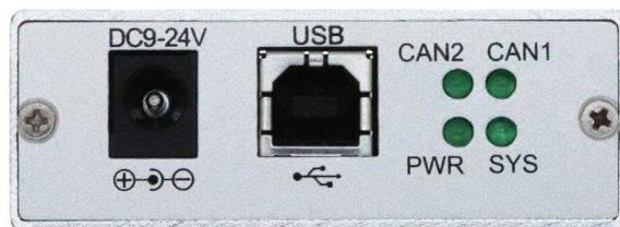
图 2.2 USB 及辅助电源接口位置
