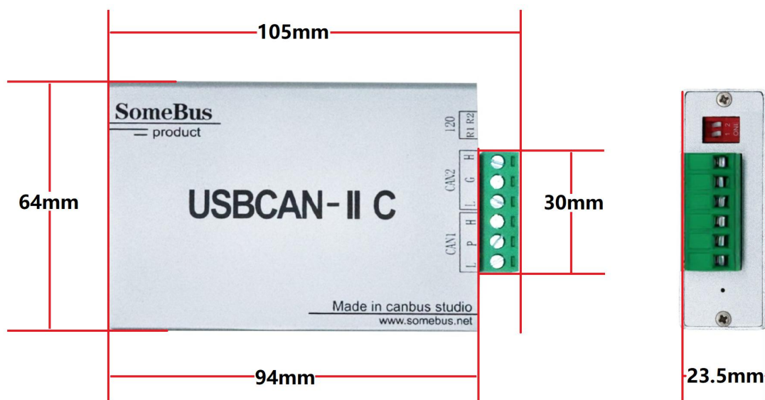
图 2.1 USBCAN-II C 外形尺寸
