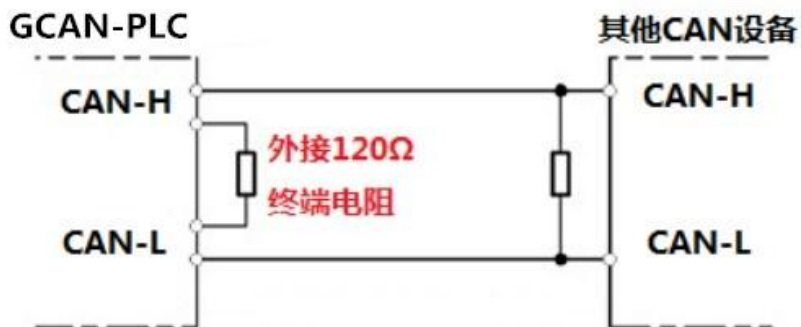
图 3.3 GCAN-PLC-220 与其他 CAN 节点设备连接
