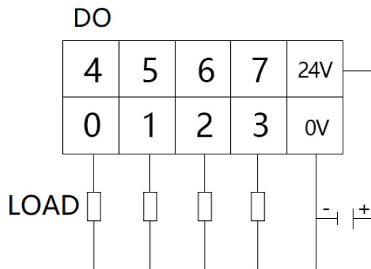
图 2.5 PLC-220 DO（0.1.2.3 路）接线
