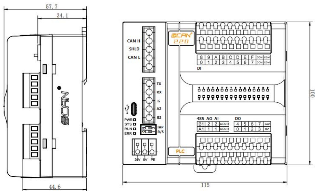
图 2.1 GCAN-PLC-220 模块外形尺寸图
