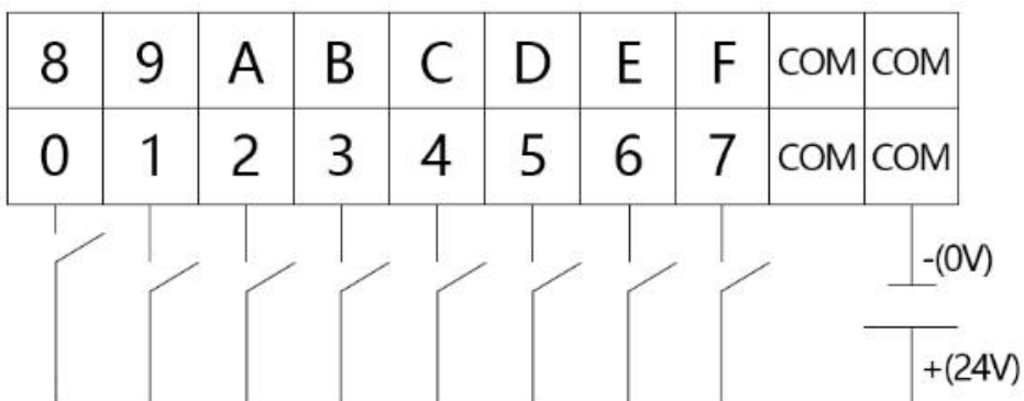
图2.7 PLC-220 DI (0-7路) 源型接线
