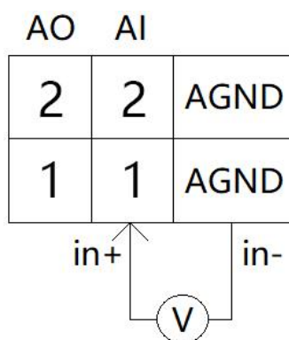
图 2.9 PLC-220 AI 接线
