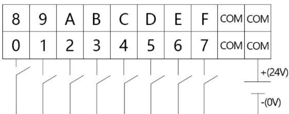
图 2.6 PLC-220 DI (0-7 路) 漏型接线
