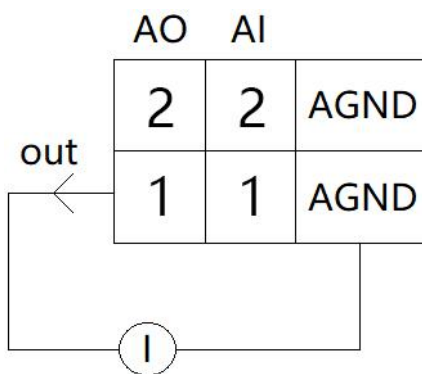
图2.8 PLC-220 AO接线
