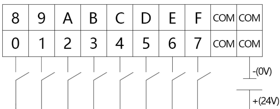
图2.9 GCAN-4032源型输入（0-7路）接线
