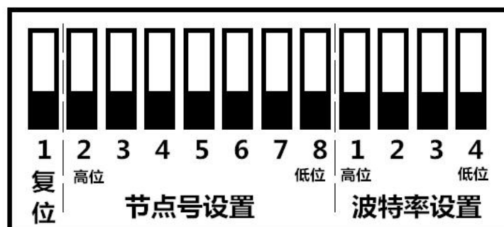
图 2.5 GCAN-4032 模块拨码开关
