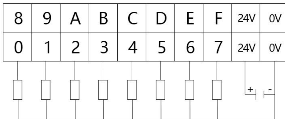
图 2.6 GCAN-4032 晶体管 PNP 输出（0-7 路）接线
