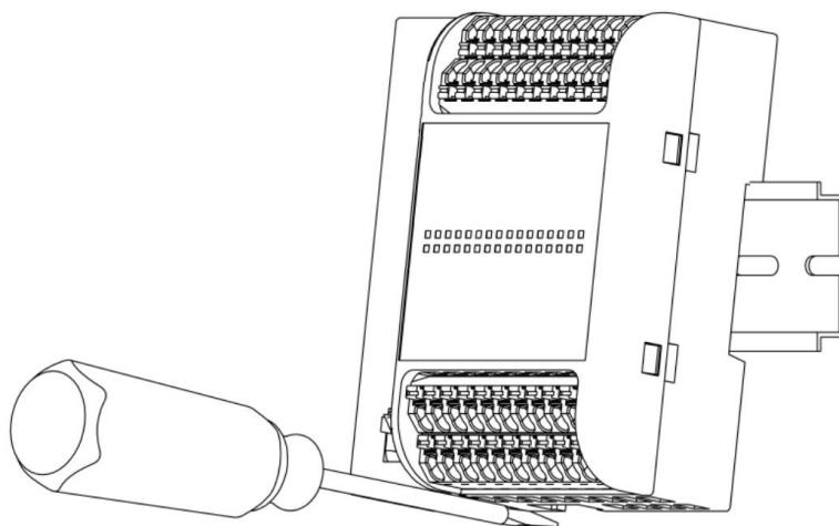
图 2.3 GCAN-4032 CANopen 模块拆卸
