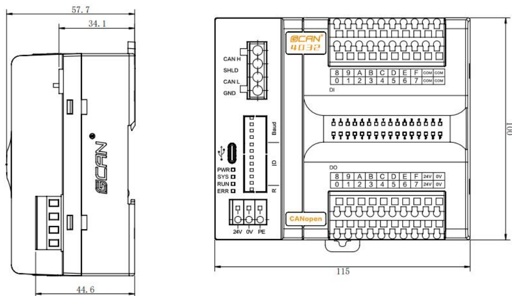
图 2.1 GCAN-4032 模块外形尺寸图
