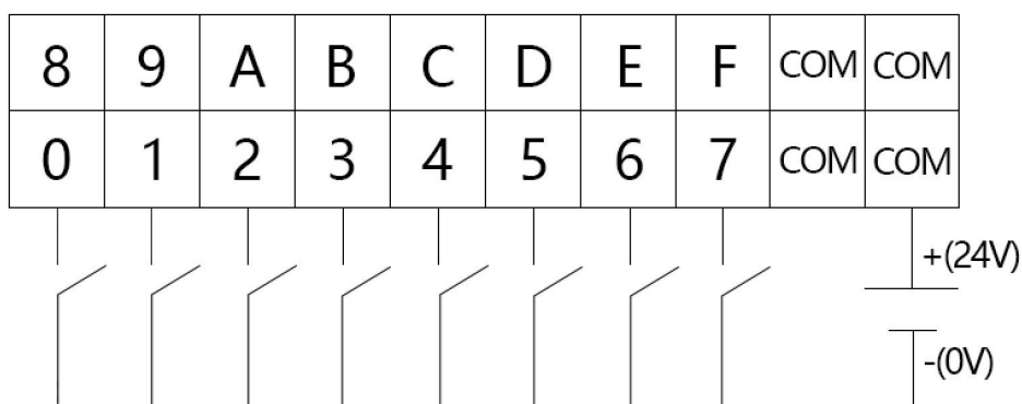
图 2.8 GCAN-4032 漏型输入（0-7 路）接线
