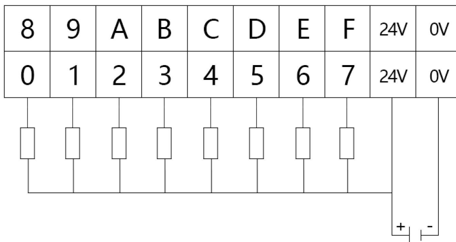
图 2.7 GCAN-4032 晶体管 NPN 输出（0-7 路）接线
