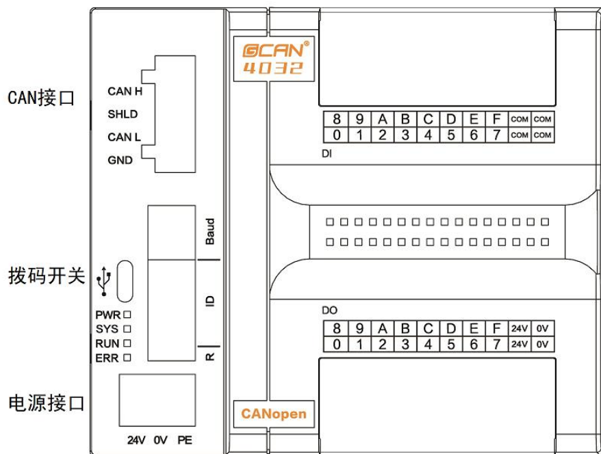
图 2.4 CAN 接口及电源接口位置
