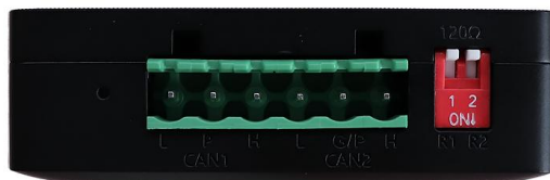
图 2.3 CAN-bus 接口位
