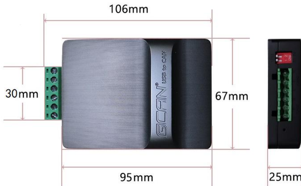
图 2.1 USBCAN-I Pro+外形尺寸
