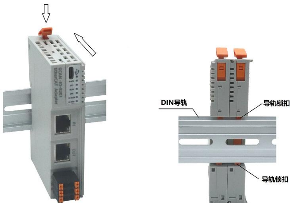
图 2.3 GCAN-PLC-425 可编程逻辑控制器模块安装
