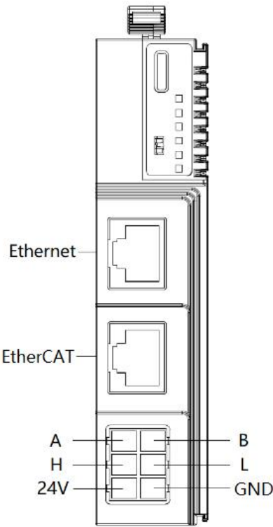
图 2.7 GCAN-PLC-425 总线及电源接线端子排
