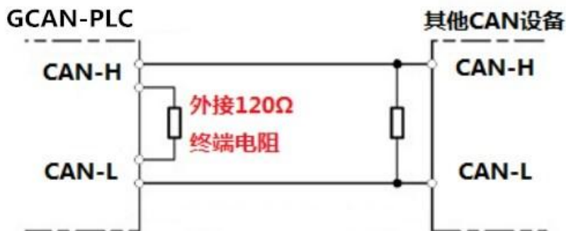
图 3.2 GCAN-PLC-425 与其他 CAN 节点设备连接
