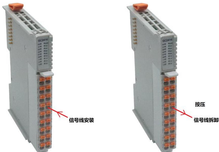
图 2.6 接线方法
