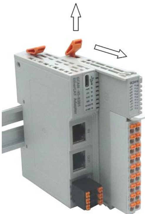
图 2.5 GCAN-PLC-425 可编程逻辑控制器拆卸
