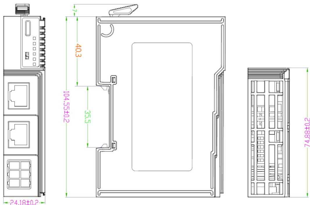
图 2.1 GCAN-PLC-425 可编程逻辑控制器外观及尺寸图
