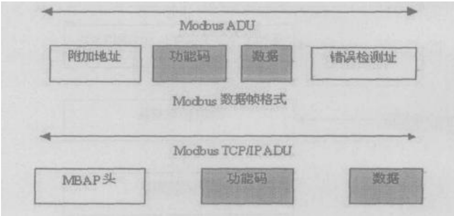
图 B.1 Modbus 与 Modbus TCP/IP 帧格式
