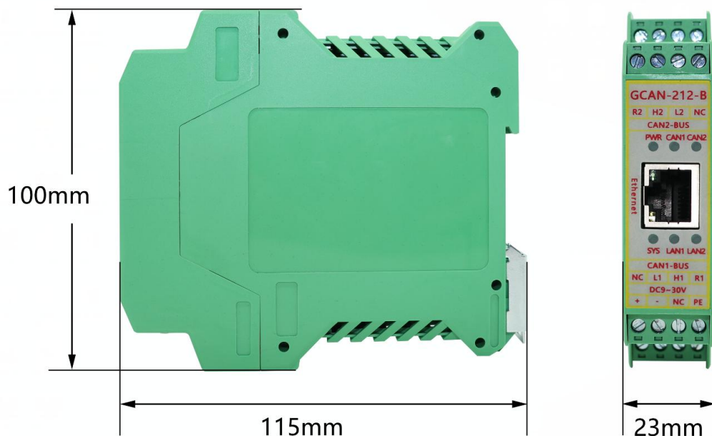
图 2.1 GCAN-212-B 模块外形尺寸
