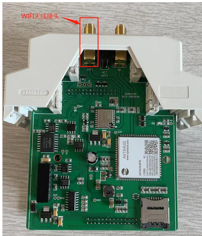
图 3.4 GCAN-GT-415 安装 WIFI 天线
