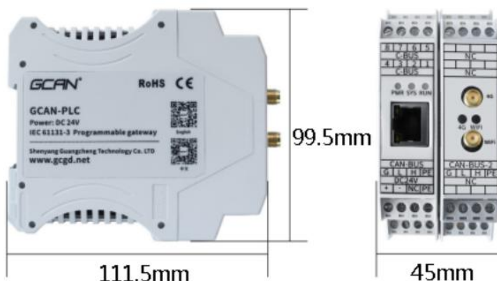
图 2.1 GCAN-GT-415 模块尺寸图
