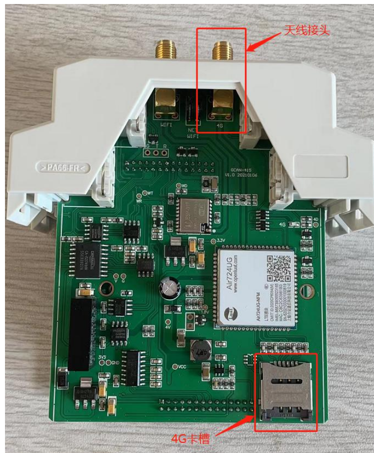
图 3.3 GCAN-GT-415 安装 4G 天线及 4G 卡位置
