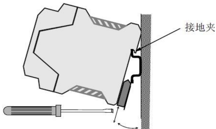
图 2.2 GCAN-GT-415 模块安装
