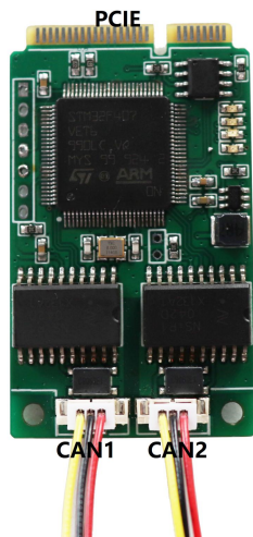
图 2.2 CAN-bus 接口、PCIE 接口位置
