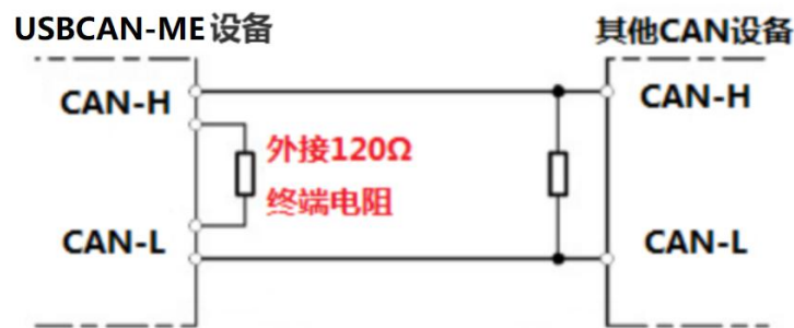
图 3.2 USBCAN-ME 与其他 CAN 节点设备连接
