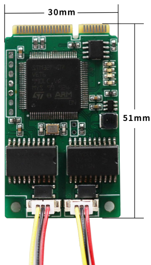
图 2.1 USBCAN-ME 外形尺寸
