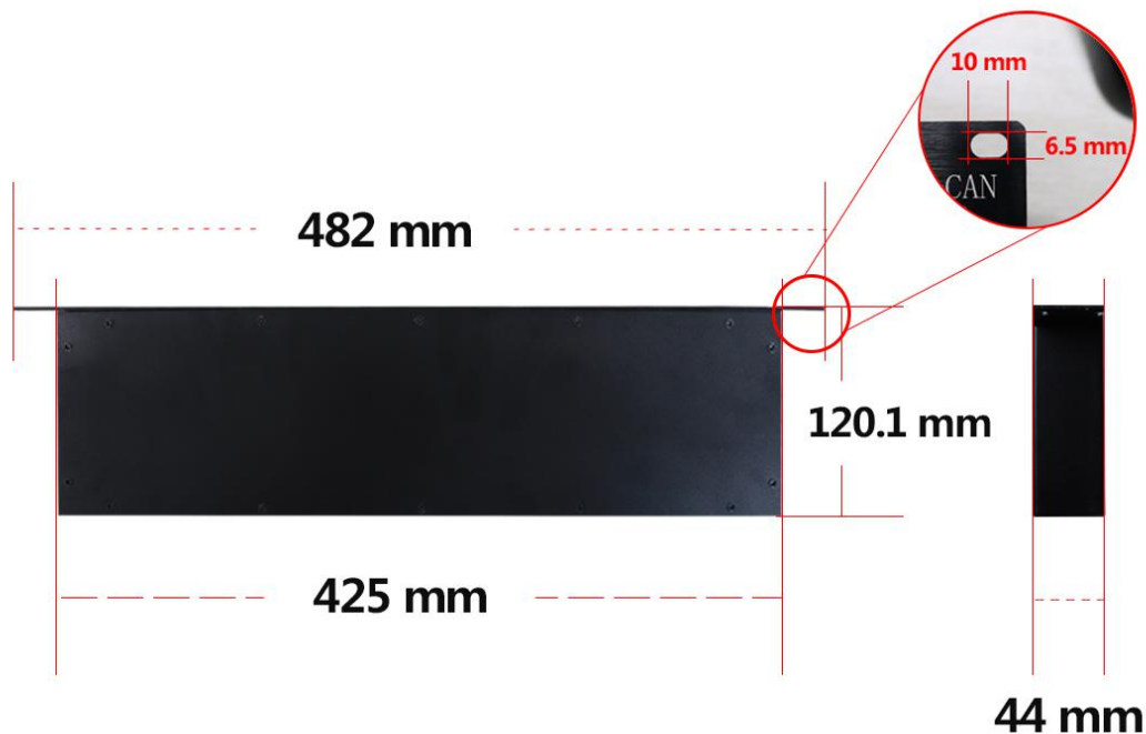
图 2.1 USBCAN-Modul 16 外形尺寸
