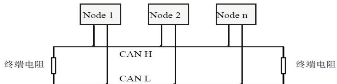
图 3.1 CAN-Bus 网络的拓扑结构
