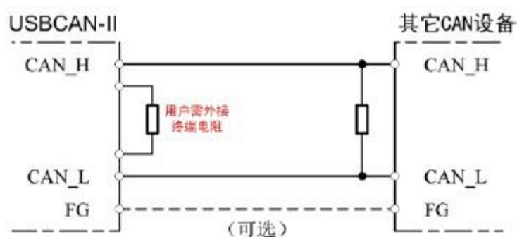
图 3.2 USBCAN-Modul 8 与其他 CAN 节点设备连接
