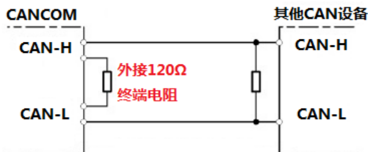
图 3.2 GCAN-207 与其他 CAN 节点设备连接
