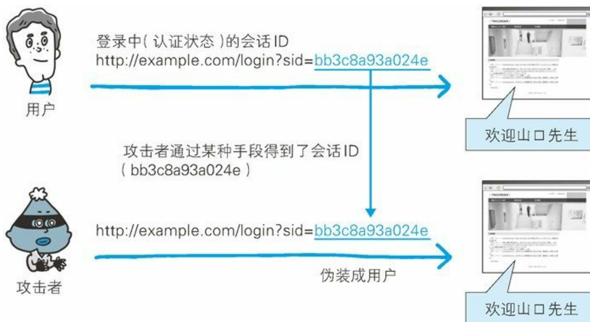
图：会话劫持
