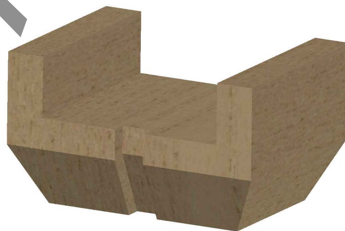
槽升子
